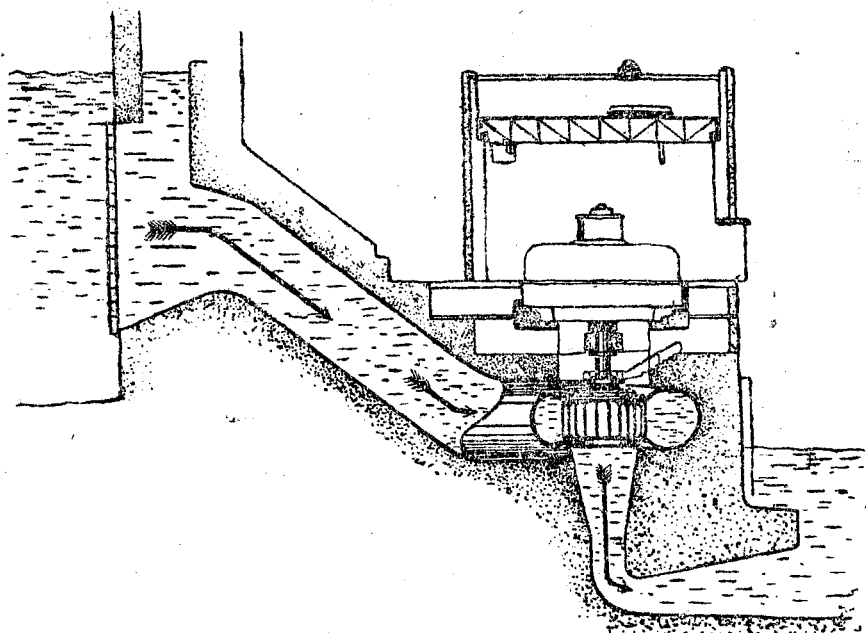
33-бд серпас. Днепрогэс вылын водяной турбиналон установка.
