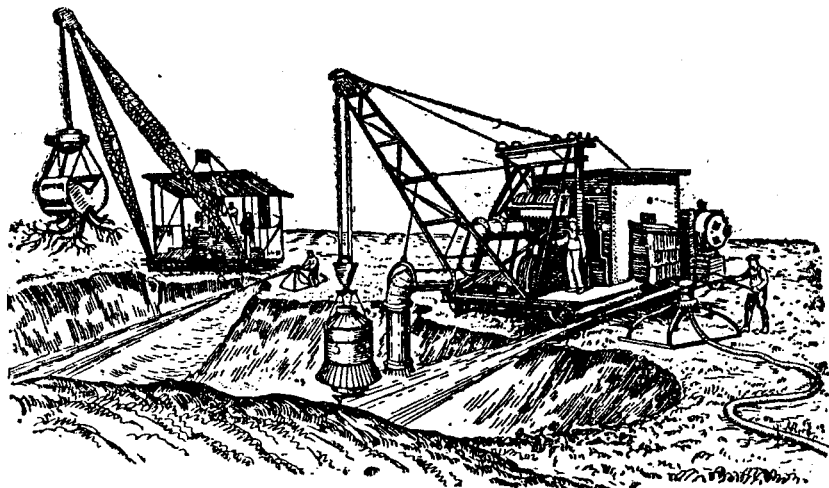
13-од серпас. Машинаясон торф перйом.
