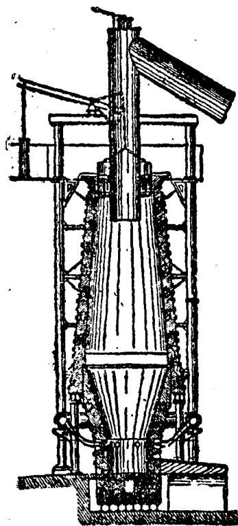
23-бд серпас. Доменнöй пач.
