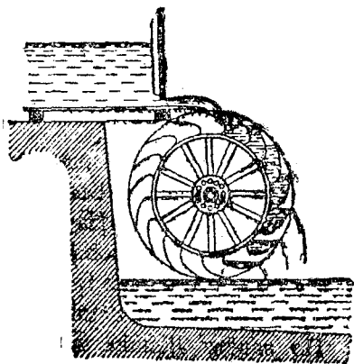
32-öд серпас. Водянöй кöлеса (наливнöй).
